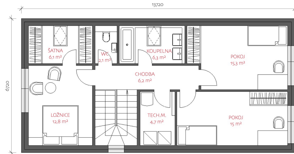
2.NP
